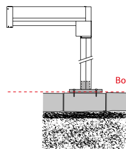
Fixation des montants sur dalles en béton ou sur fondations
