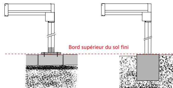
Fixation des montants sur dalles en béton ou sur fondations
