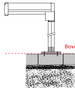
Bevestiging van de staanders op betonnen bodemplaten of fundering
